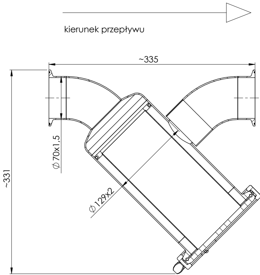
PRZEKRÓJ A-A
