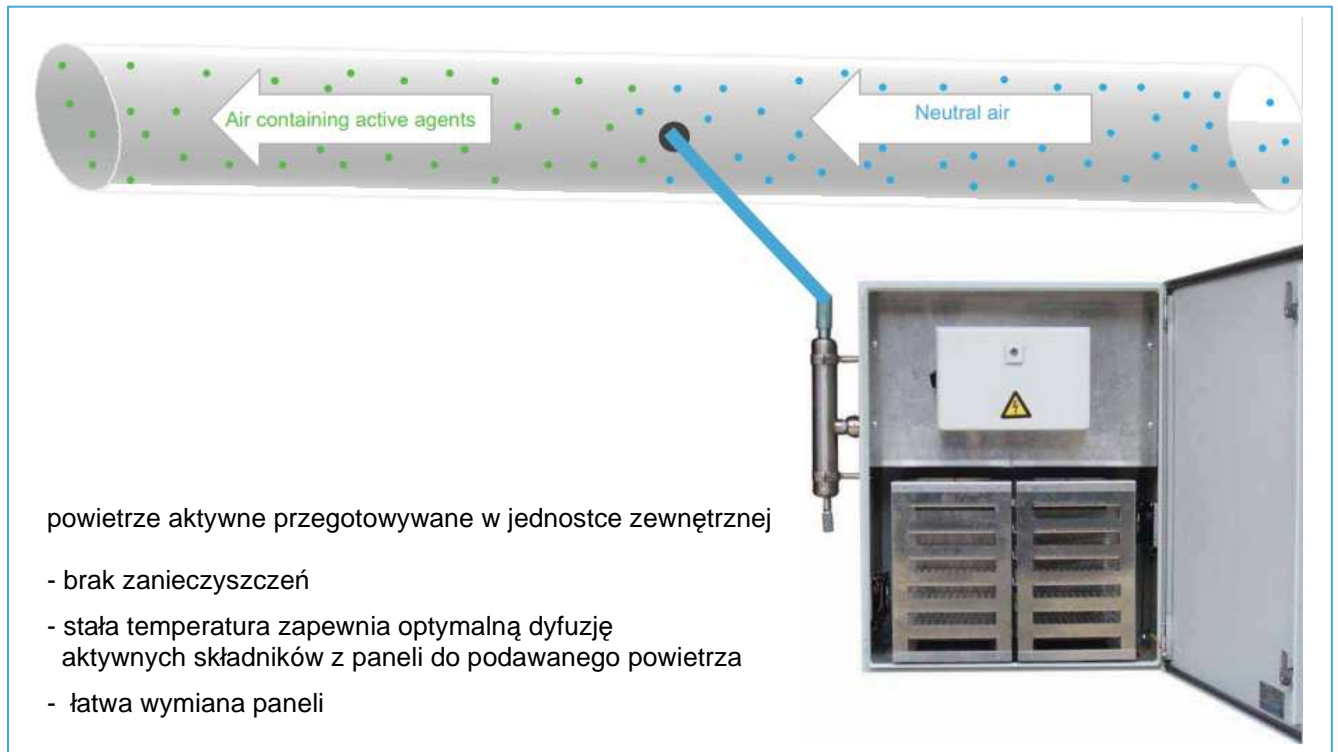
aplikacja do kanału wentylacyjnego
